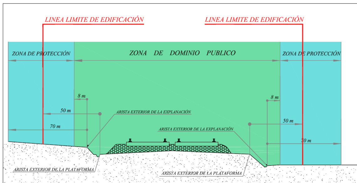
Croquis de Dominio Público y Afecciones Líneas de Ferrocarril, según establece la Ley 38/2015, de 29 de septiembre, del Sector Ferroviario.
