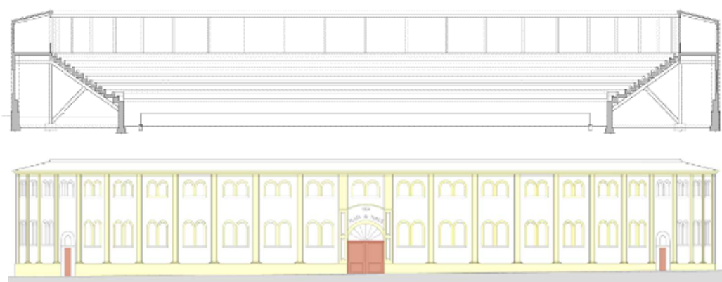
Sección y Alzado. Estado actual
